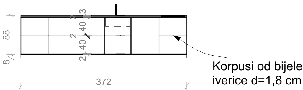
presjek podužni
